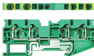
DST 4/4-PE-D
